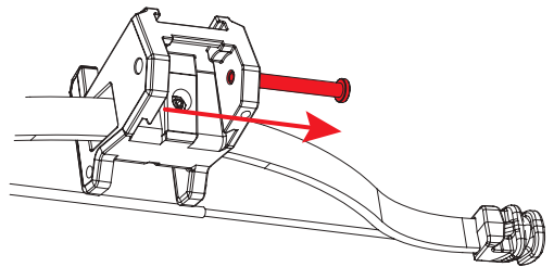
Schnellverschlussstifte
